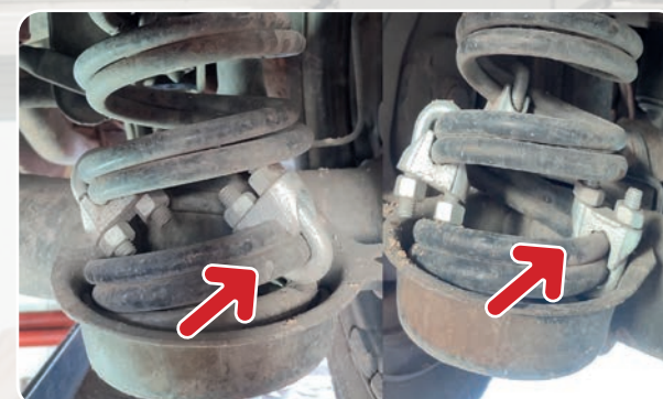
EJES, RUEDAS, NEUMÁTICOS Y SUSPENSIÓN Muelle de suspensión reforzado caseramente
